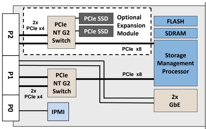
StoreEngine SE300-CCVPX Diagram.
